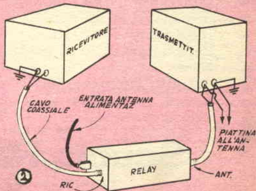
Scheda indicante le connessioni esterne, in partenza ed arrivo al complesso.
